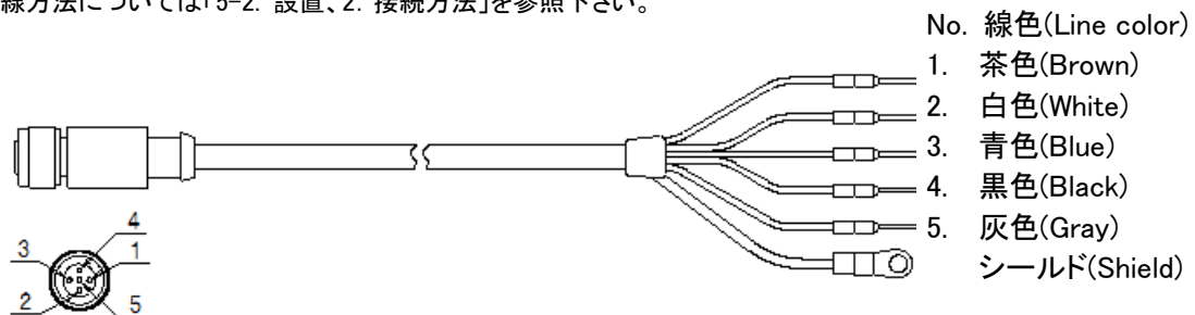
図 7-2. 出カケーブル
