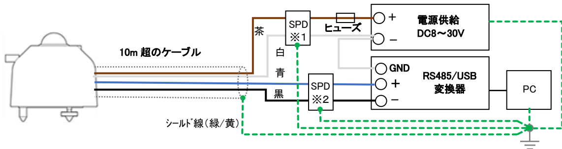
図 A9-1. Modbus RTU 接続(ケーブル長が 10m を超える場合等)
