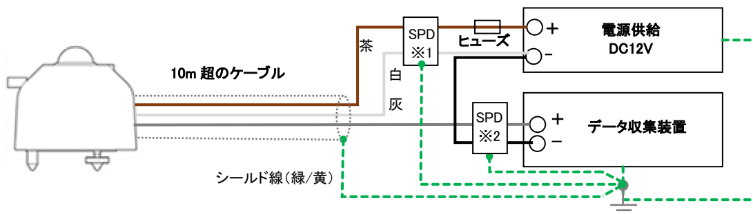
図 A9-3.SDI-12 接続(ケーブル長が 10m を超える場合等)
