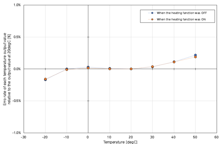
図 A6-1. ドームヒーティング機能 ON 時と OFF 時の温度特性結果比較
