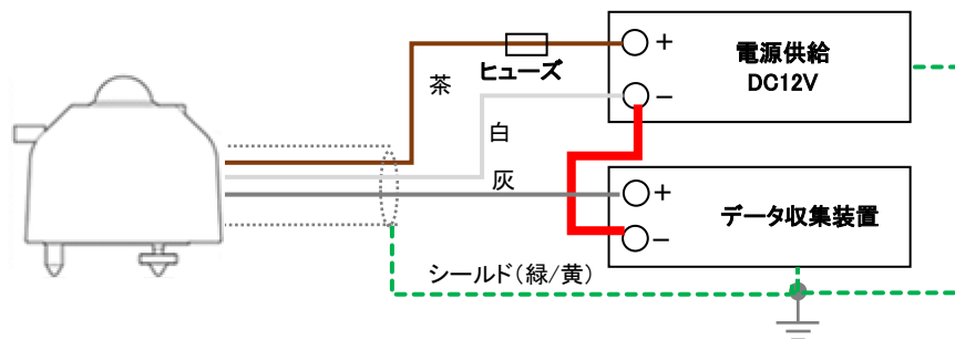
図 5-7b. MS-80SH の SDI-12 の接続方法 (S23038501 以降の MS-80SH)
