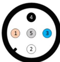
図 5-9. MS-80SH のコネクタピン番号
