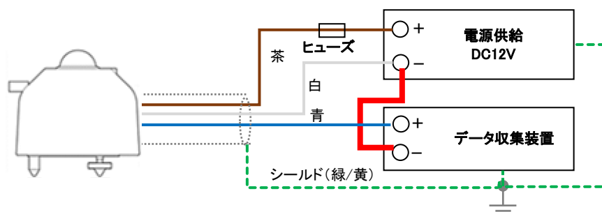
図 5-7a. MS-80SH の SDI-12 の接続方法 (S23038500 以前の MS-80SH)
