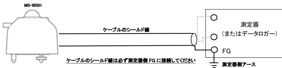
図 5-3. MS-80SH のケーブルシールド線接続方法
