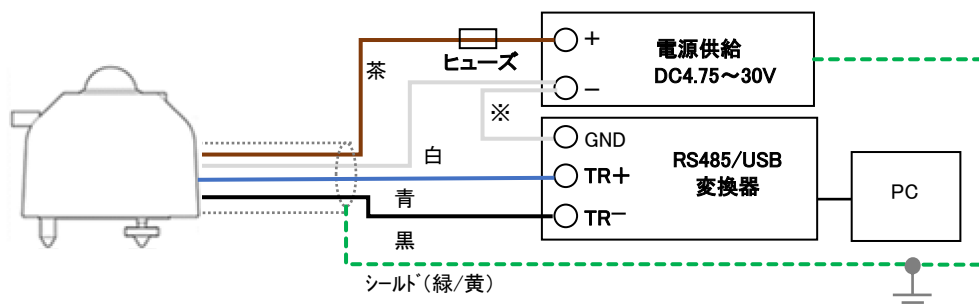
図 5-10. MS-80S の Modbus RTU 接続方法(PC)
