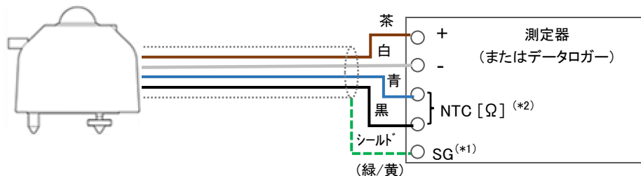
図 5-6. MS-80 の接続方法 (S19046150 以前)
