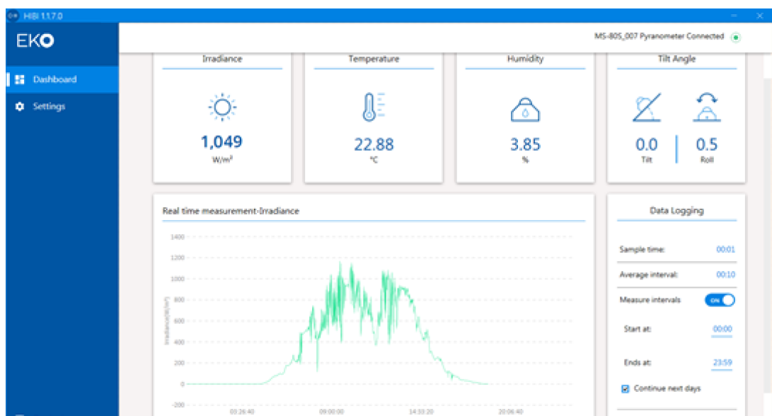
図 A3-7. 「Dashboard」画面
