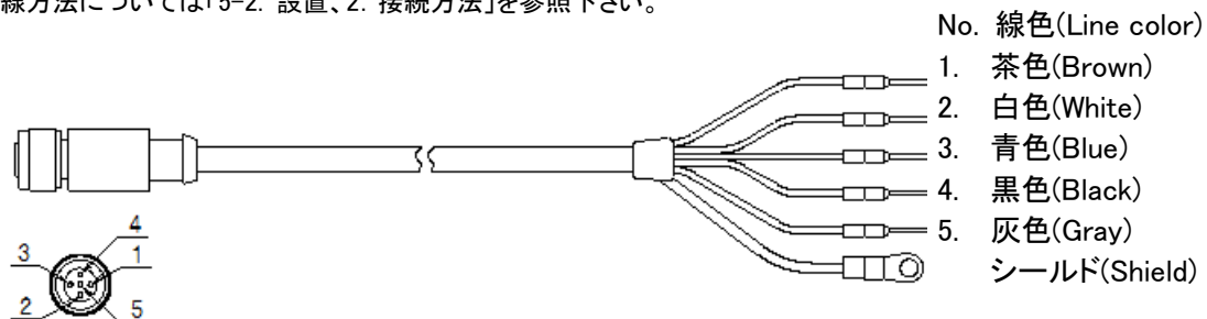
図 7-3. 出力ケーブル (MS-80 / 80S)
