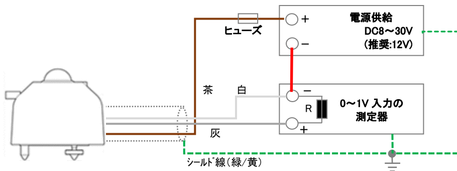
図 5-9. MS-80S の接続方法
