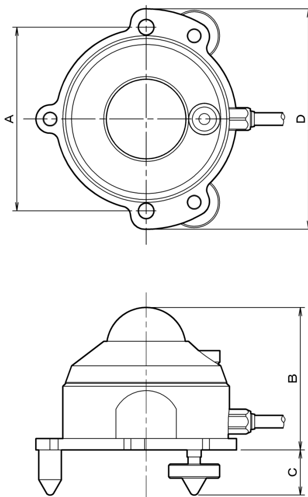
図 7-2. 外形図 (MS-80U)
