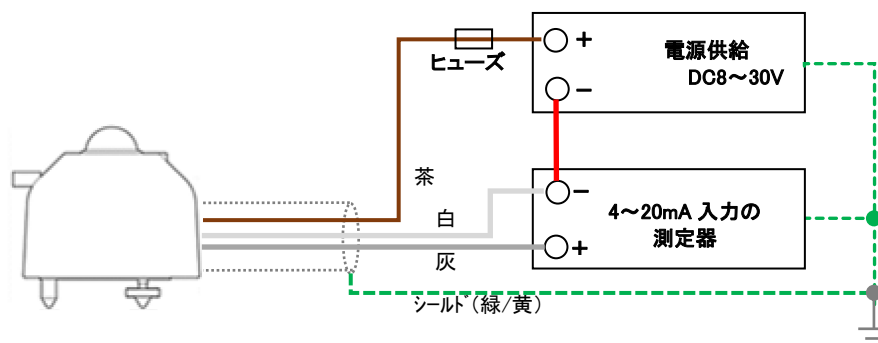
図 5-8. MS-80S の接続方法
