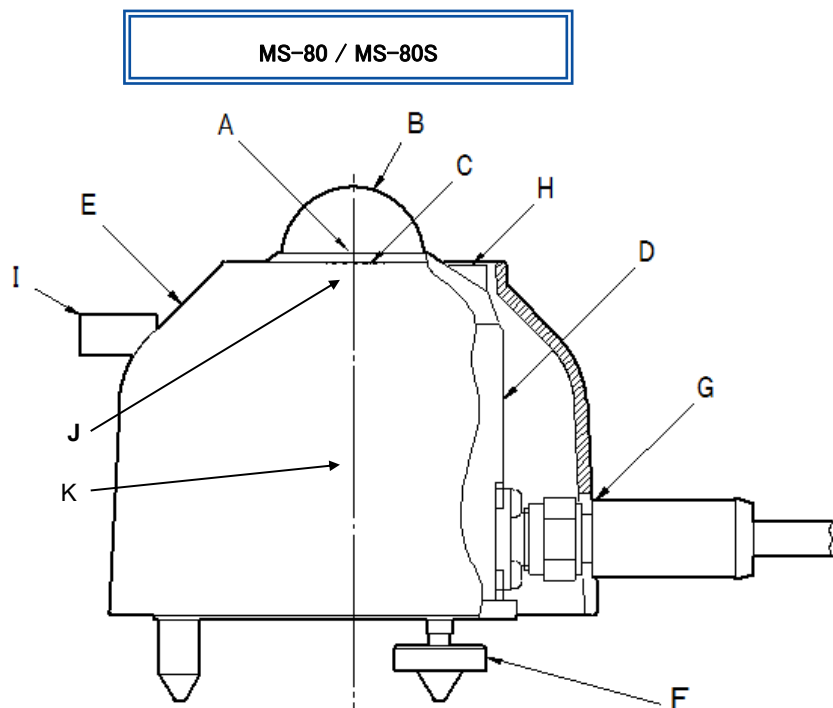
*MS-80S はボディ内部に信号変換器が内蔵されています 図 5-1. 各部名称(MS-80 / MS-80S)
