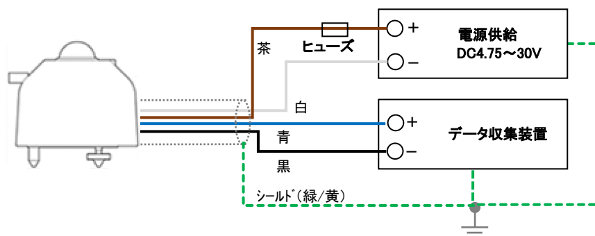
図 5-11. MS-80S の Modbus RTU 接続方法(データ収集装置)
