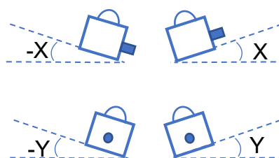
図 5.3A チルト(X 軸) (-180° to 0) と (0 to 180°) ロール(Y 軸) (-180° to 0) と (0 to 180°)
