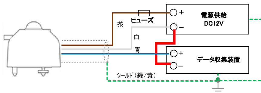
図 5-13. MS-80S の SDI-12 の接続方法
