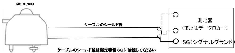
図 5-4A. MS-80/80U のケーブルシールド線接続方法
