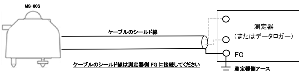
図 5-4B. MS-80S のケーブルシールド線接続方法
