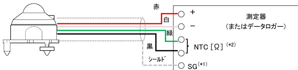
図 5-7. MS-80U の接続方法
