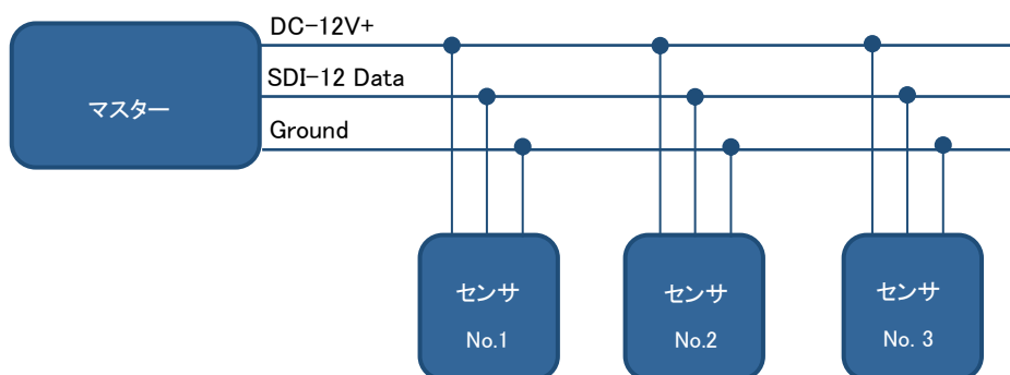
図 5-14. SDI-12 での通信接続
