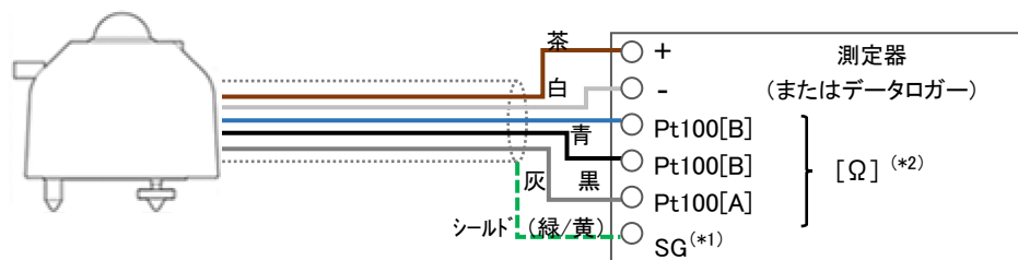
図 5-5. MS-80 の接続方法 (S19046151 以降)
