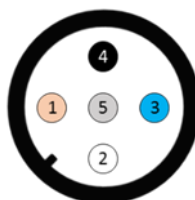
図 5-15. MS-80 および MS-80S のコネクタピン番号
