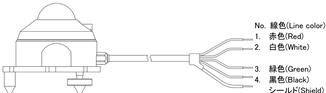
図 7-5. 出力ケーブル (MS-80U)
