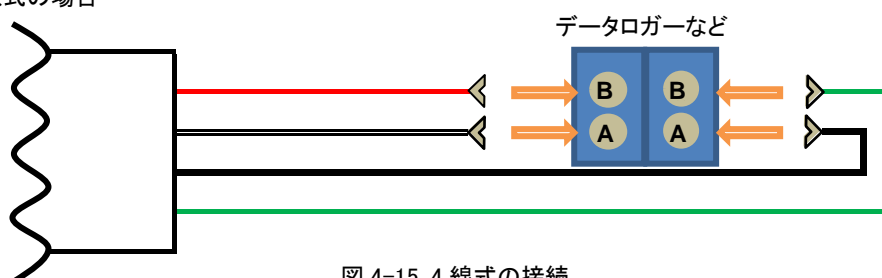
図 4-15. 4 線式の接続
