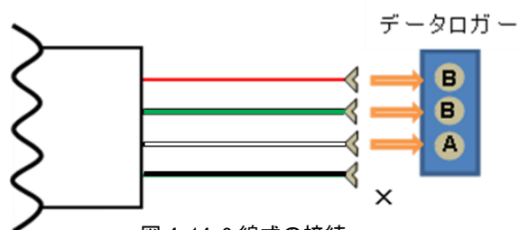
図 4-14. 3 線式の接続
