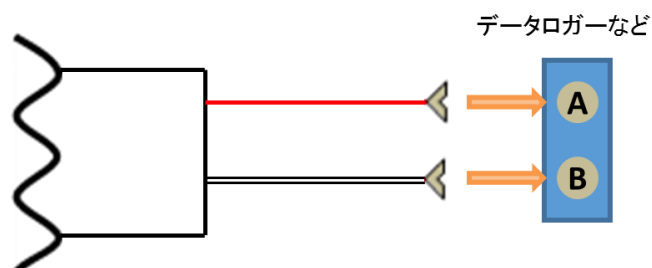
図 4-17. MT-052-T の接続例
