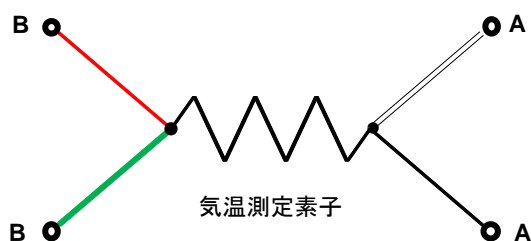
図 4-12. 気温測定素子の簡易回路
