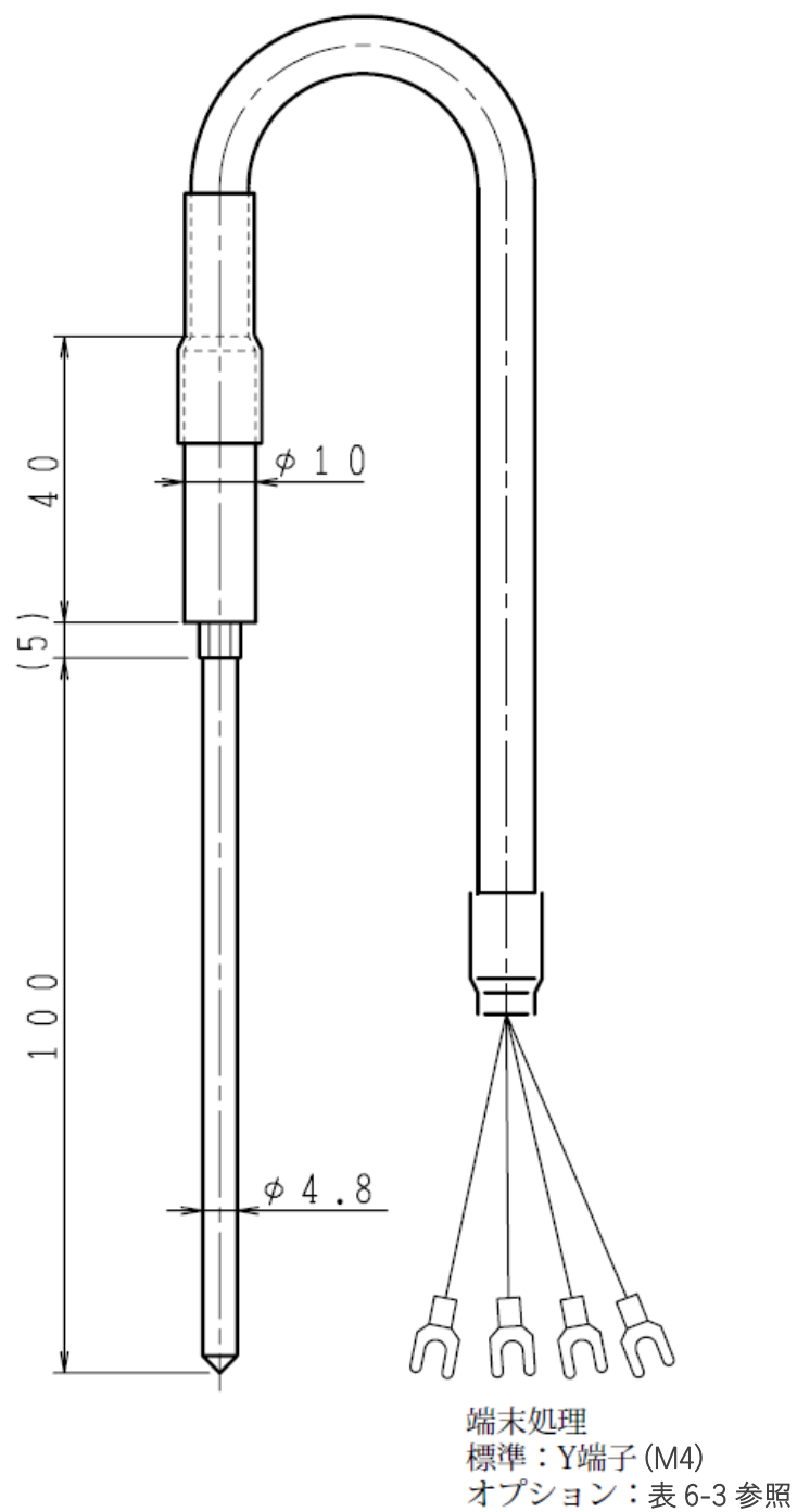
図 6-2. 気温測定素子 (MT-010-A) 寸法図
