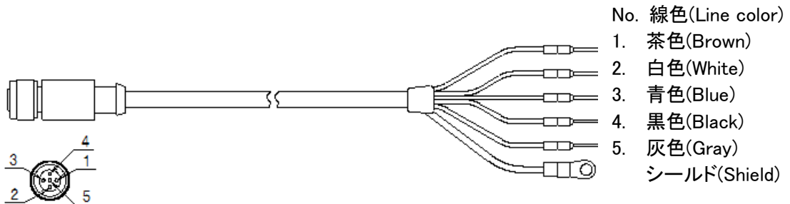
図 3-3. 出力ケーブル (MS-60S)
