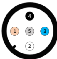
図 3-5. MS-60S のコネクタピン番号
