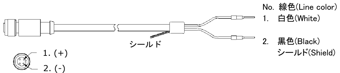
図 3-2. 出力ケーブル (MS-60)
