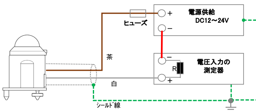
図 5-5. MS-60A の接続方法
