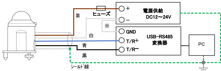
図 5-6. MS-60M の Modbus RTU 接続方法(PC)
