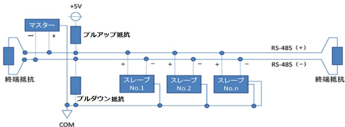
図 5-8. MS-60M の接続方法
