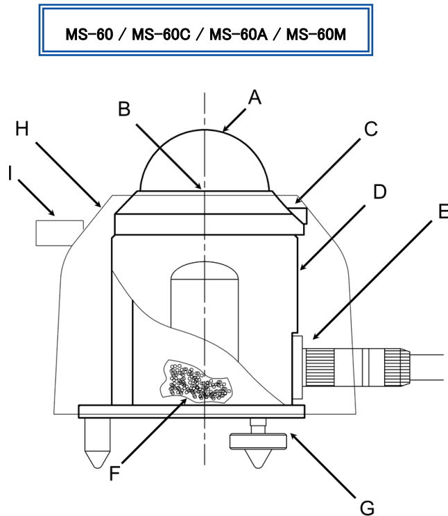
図 5-1. 各部名称
