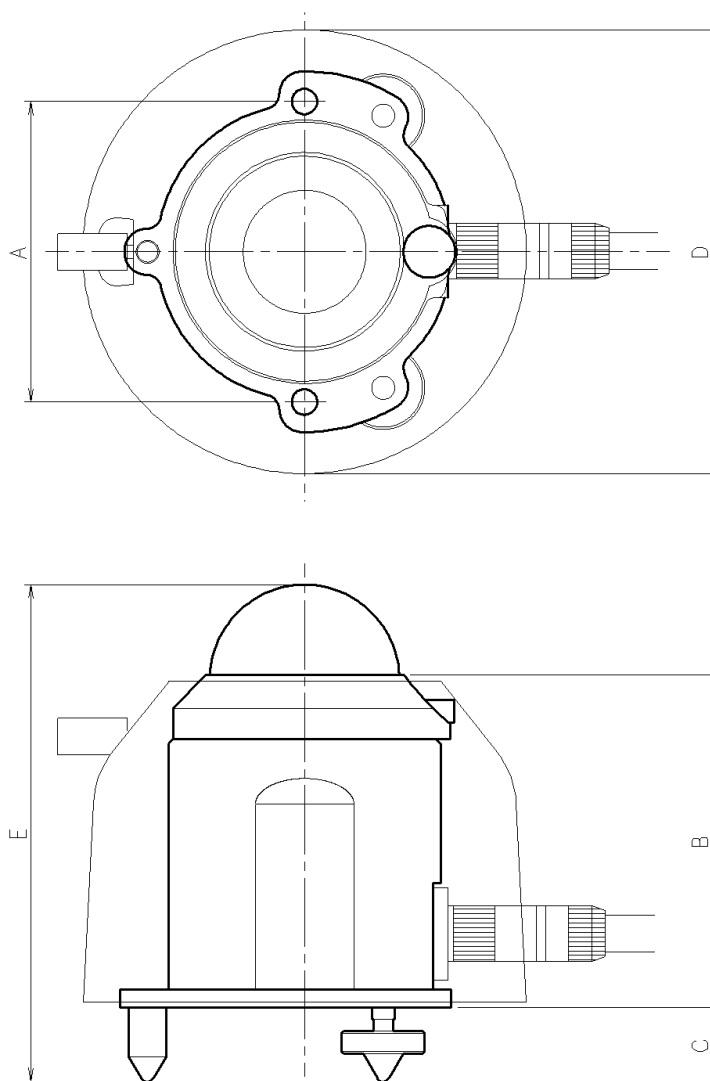
図 7-1. 外形図
