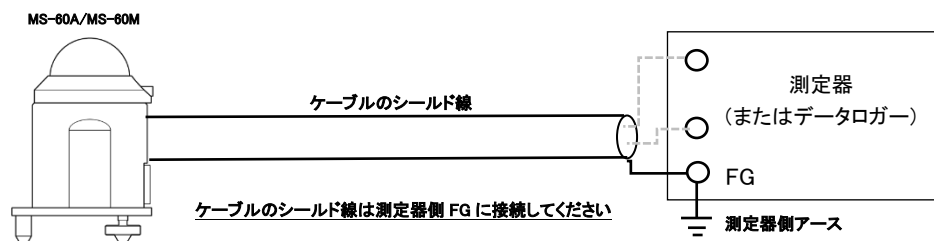
図 5-3. MS-60A/MS-60M のケーブルシールド線接続方法
