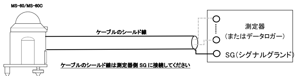
図 5-2. MS-60/MS-60C のケーブルシールド線接続方法
