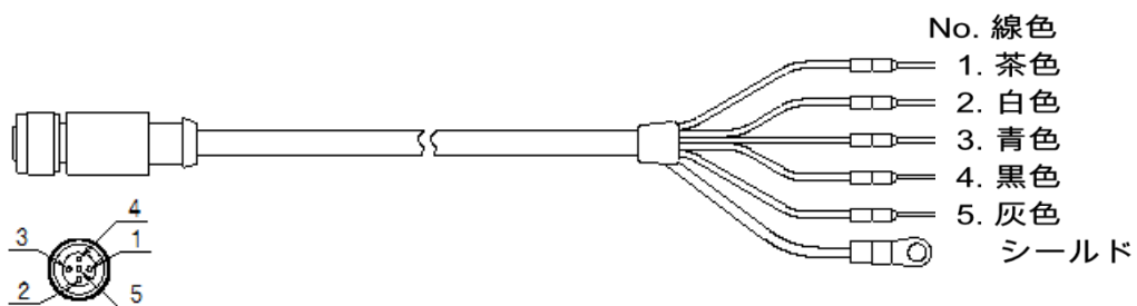
図 7-4. 出力ケーブル (MS-60A、MS-60M)
