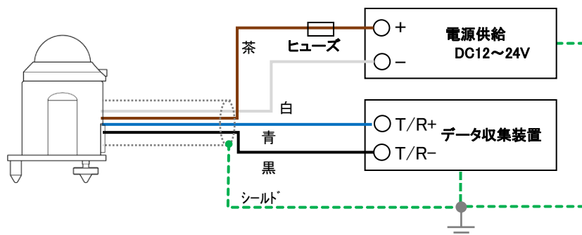
図 5-7. MS-60M の Modbus RTU 接続方法(データ収集装置)
