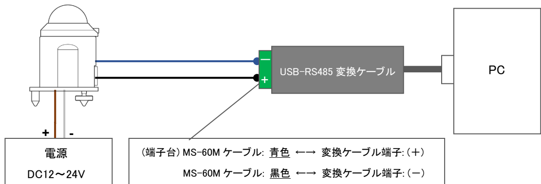
図 A-6. USB-RS485 変換ケーブルでの接続方法
