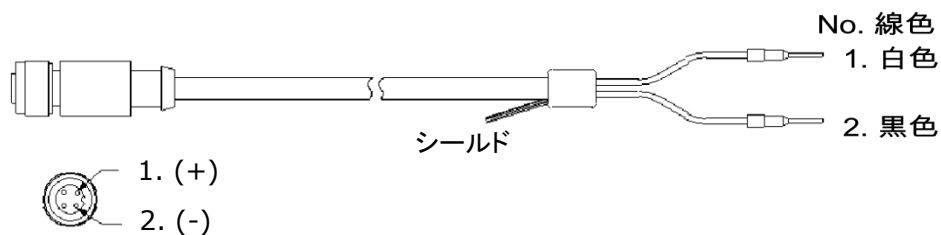
図 7-2. 出力ケーブル (MS-60)
