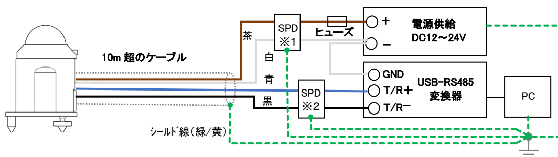
図 A6-1. Modbus 接続(ケーブル長が10mを超える場合等)
