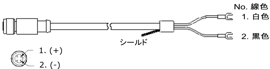
図 7-3. 出力ケーブル (MS-60C)
