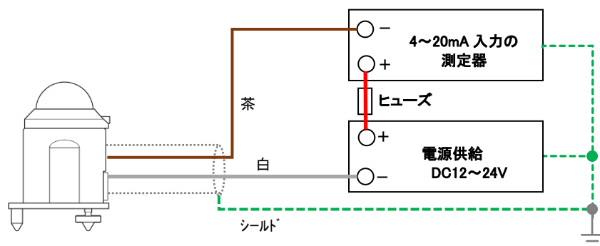
図 5-4. MS-60A の接続方法
