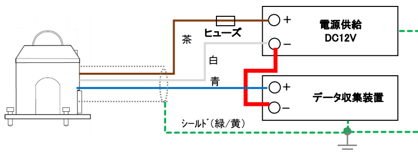
図 5-9. MS-40S の SDI-12 の接続方法
