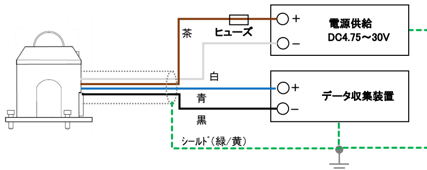
図 5-7. MS-40S の Modbus RTU 接続方法(データ収集装置)
