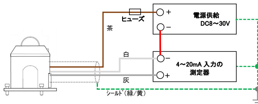
図 5-4. MS-40S の接続方法
