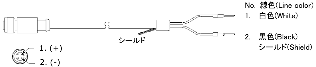
図 7-2. 出力ケーブル (MS-40)
