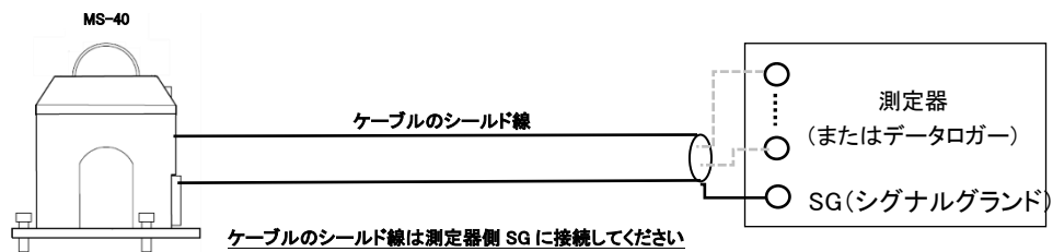
図 5-3A. MS-40 のケーブルシールド線接続方法
