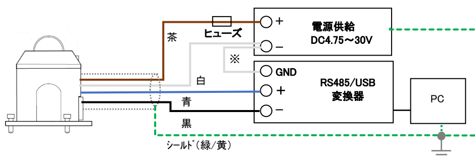
図 5-6. MS-40S の Modbus RTU 接続方法(PC)
