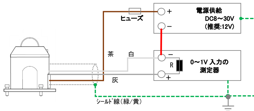
図 5-5. MS-40S の接続方法
