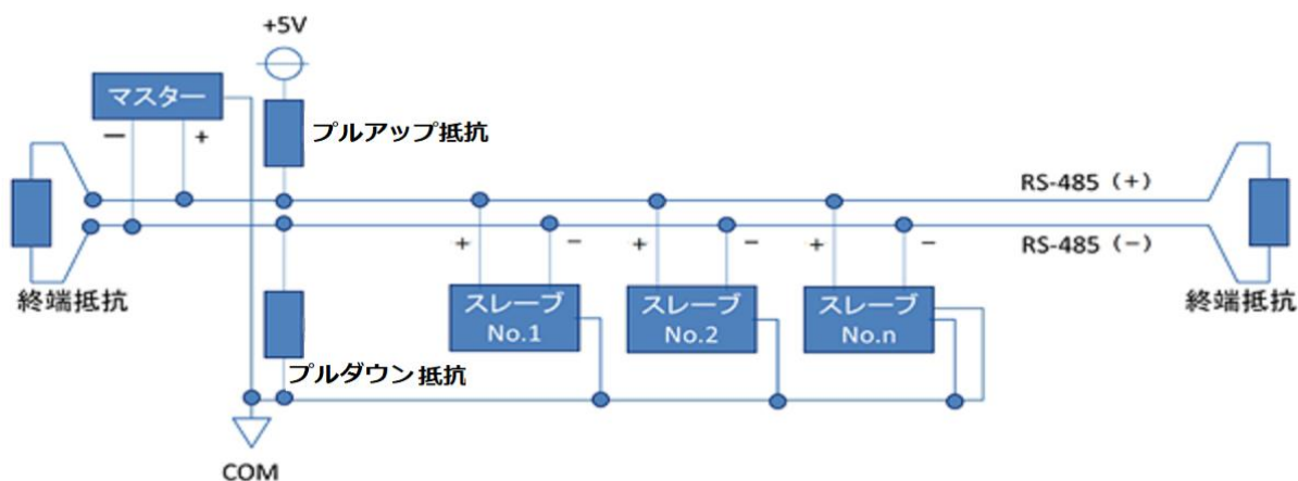
図 5-8. MS-40S の接続方法
