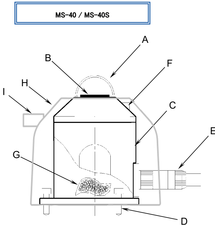
図 5-1. 各部名称(MS-40 / MS-40S)
