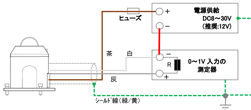
図 5-6. MS-40S の接続方法 (0-1V)
