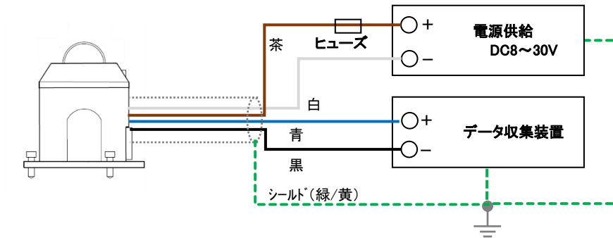
図 5-8. MS-40S の Modbus RTU 接続方法(データ収集装置)
