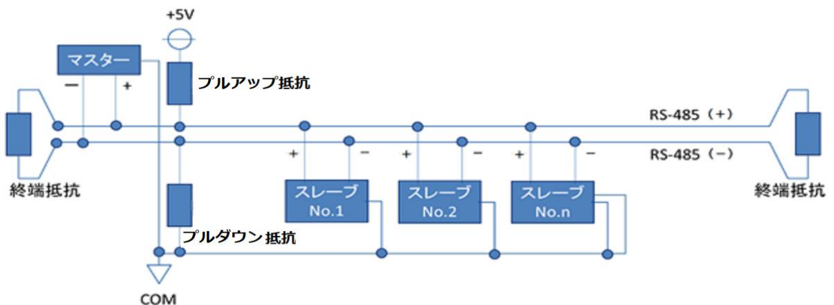
図 5-9. MS-40S の接続方法
