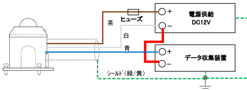
図 5-10. MS-40S の SDI-12 の接続方法
