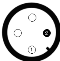
図 5-12. MS-40/MS-40C のコネクタピン番号
