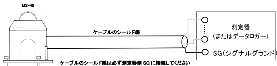
図 5-3A. MS-40/MS-40C のケーブルシールド線接続方法
