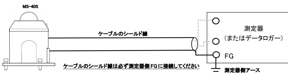
図 5-3B. MS-40S のケーブルシールド線接続方法
