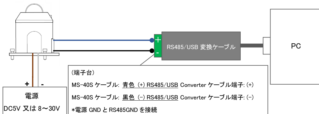
図 A3-1. ハードウェアの準備
