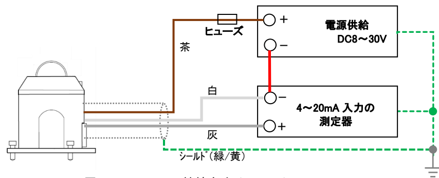
図 5-5. MS-40S の接続方法 (4-20mA)
