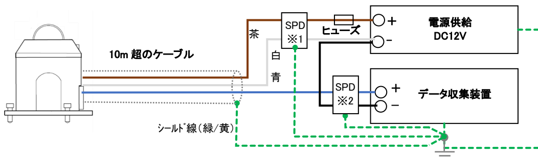
図 A8-2. SDI-12 接続(ケーブル長が 10m を超える場合等)
