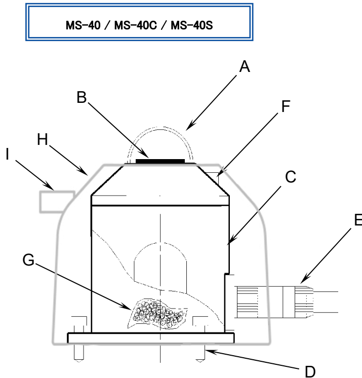
*MS-40S はボディ内部に信号変換器が内蔵されています 図 5-1. 各部名称(MS-40 / MS-40C / MS-40S)
