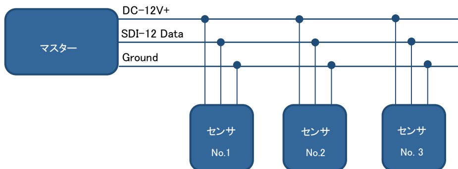
図 5-11. SDI-12 での通信接続
