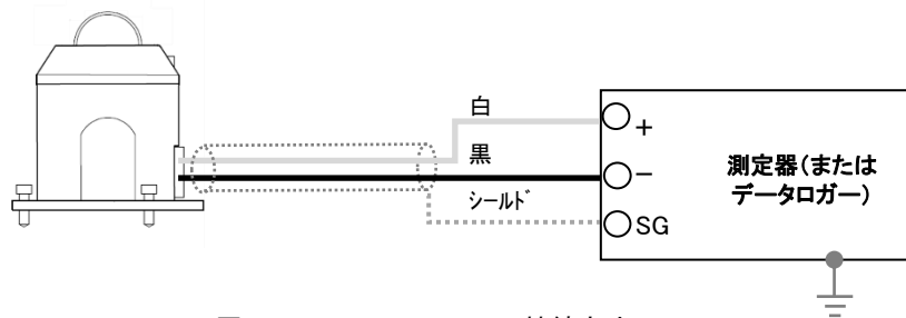
図 5-4. MS-40, MS-40C の接続方法
