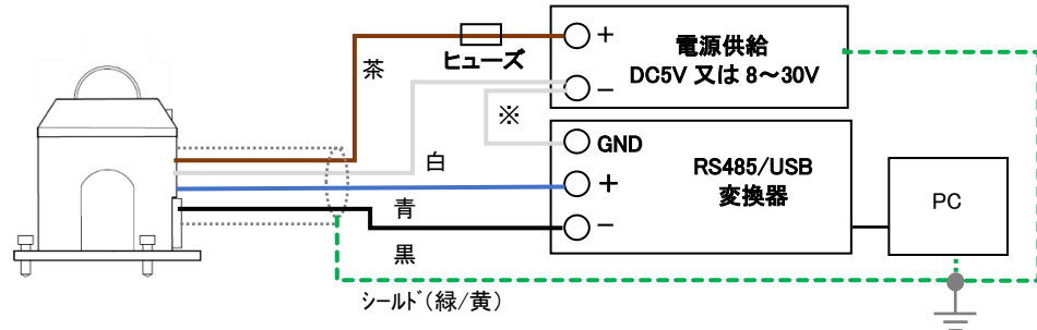
図 5-7. MS-40S の Modbus RTU 接続方法(PC)
