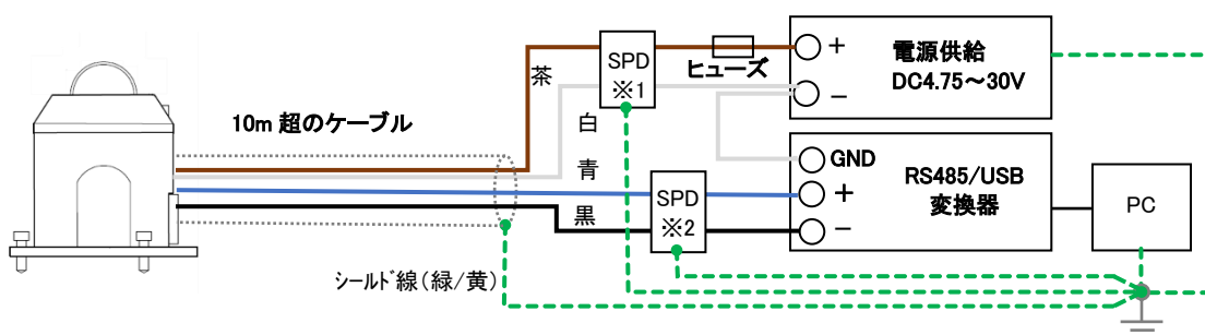
図 A8-1. Modbus RTU 接続(ケーブル長が 10m を超える場合等)
