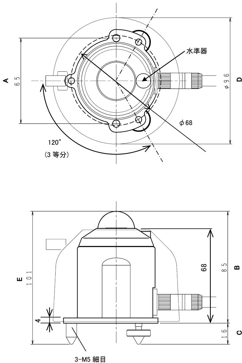
図 3-2. 外形図
