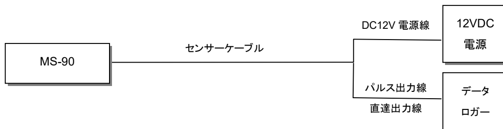
図 5-4. 接続方法
