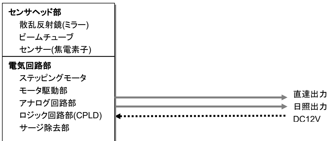
図 5-2. 構成図
