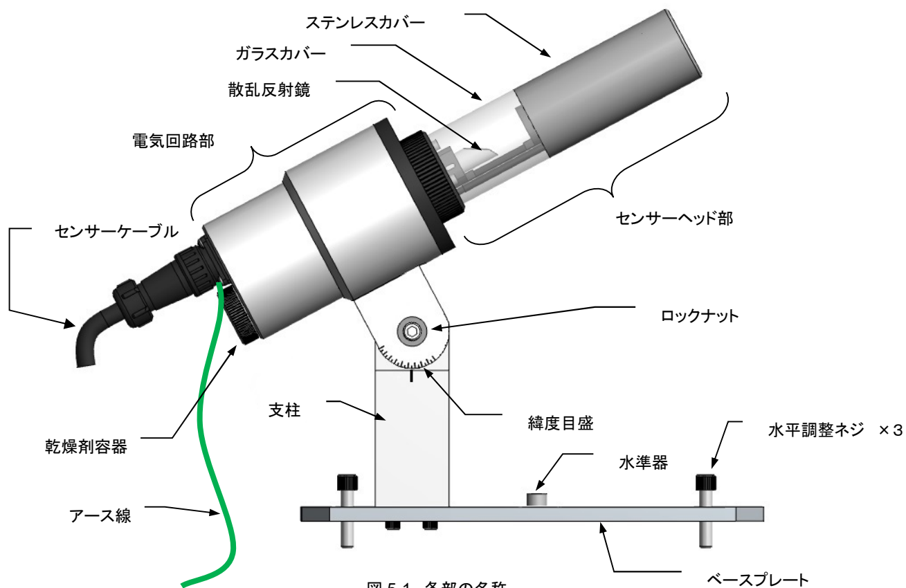
図 5-1. 各部の名称
