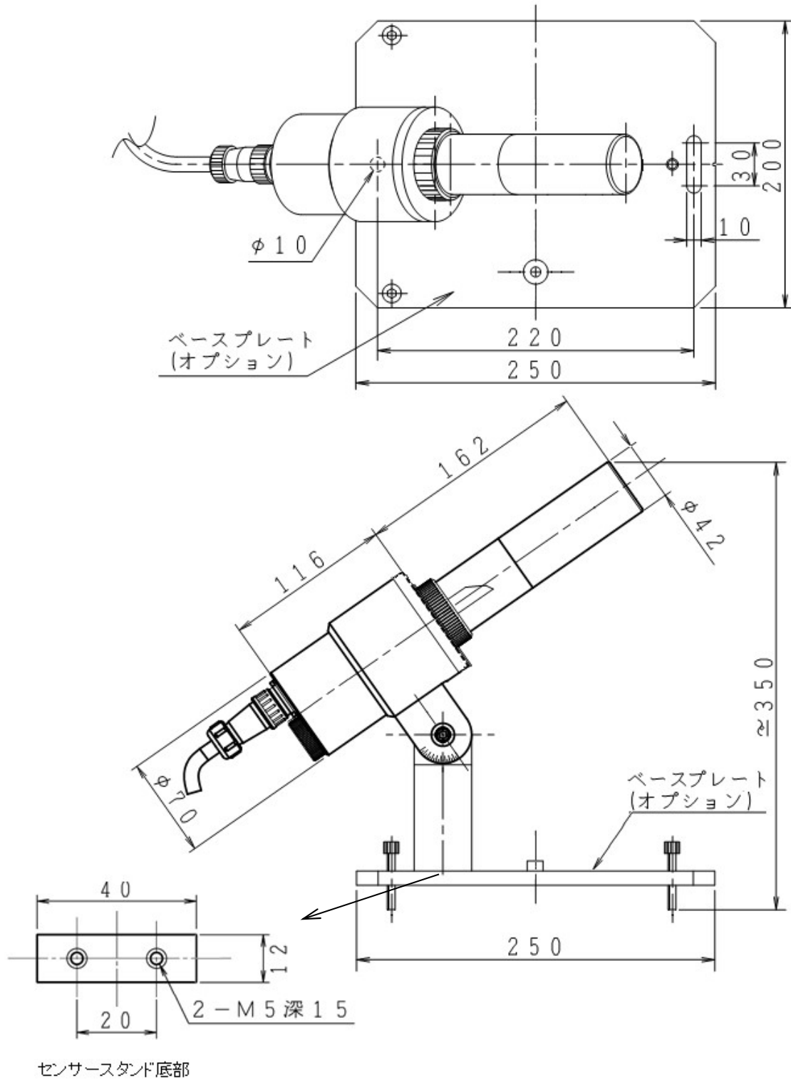
図 8-2. MS-90 寸法図
