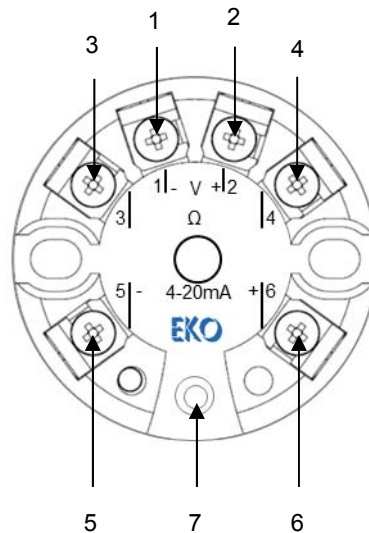
図 5-1. 各部の名前
