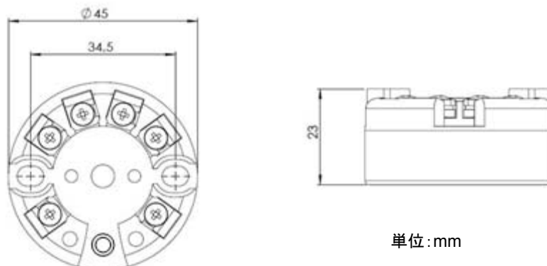
図 7-1. 寸法図
