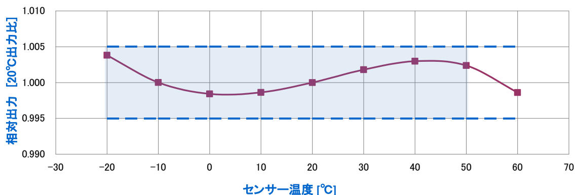
図 7-2. 温度特性測定(例)
