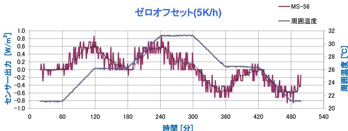
図 7-3. ゼロオフセット測定(例)
