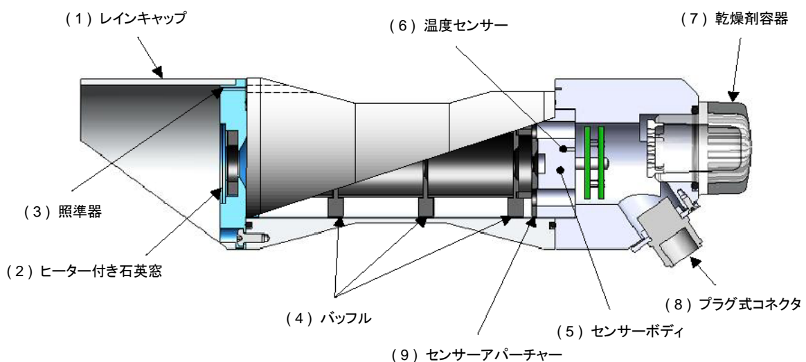
図 5-1. MS-56 本体
