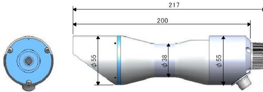
図 7-1. MS-56 寸法図
