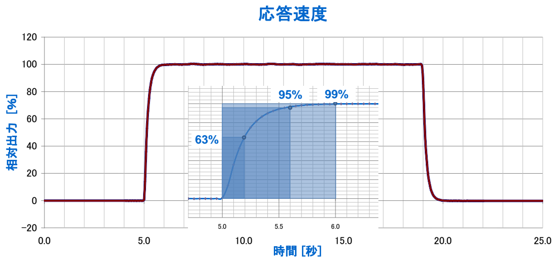
図 7-1. 応答速度測定(例)
