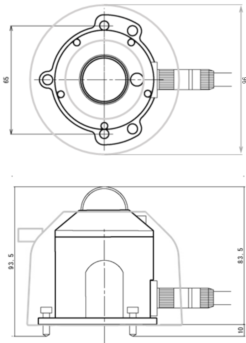
図 7-1. 外形図
