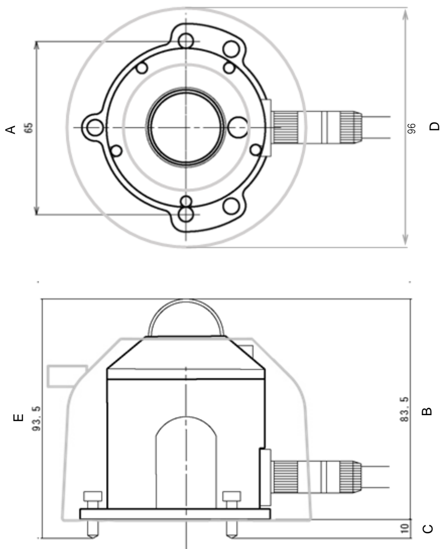
図 7-1. 外形図
